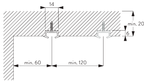
Nut Kanal: 6 x 14 mm
